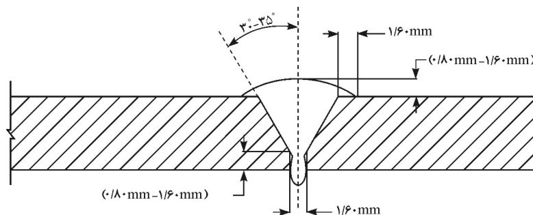
شکل ۱۷- ۵- ۶- ۲ طرح اتصال جوش لب به لب.
