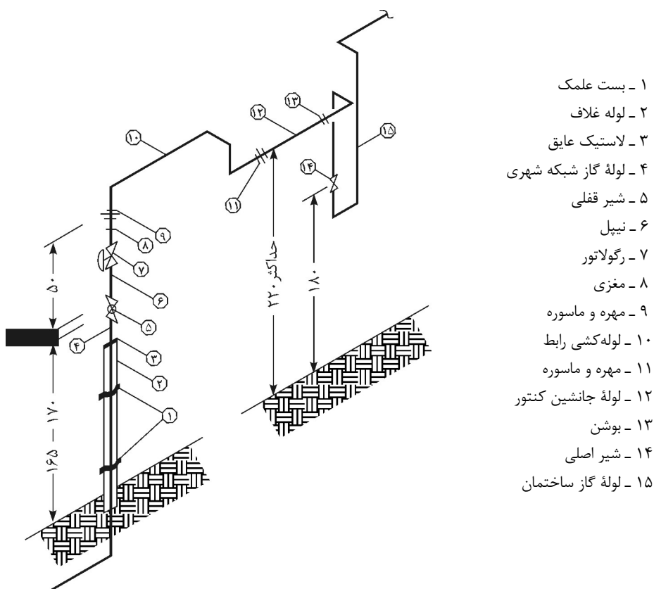
شکل ۱۷- ۴- ۲- ۱ نمونه تعیین محل نصب کنتور گاز و لوله رابط.
